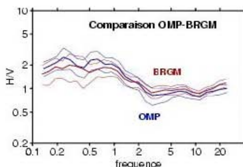
Fig. 3. Comparaison des rapports H/V obtenus par le BRGM et l'OMP avec une série commune de mesures d'inter-calibration à Toulouse le 15/03/2005 (données BRGM communiquées par A. Roullé). On note que la cohérence est aussi bonne que dans le cas des Fig. 1 et 2, où les appareils sont identiques.
