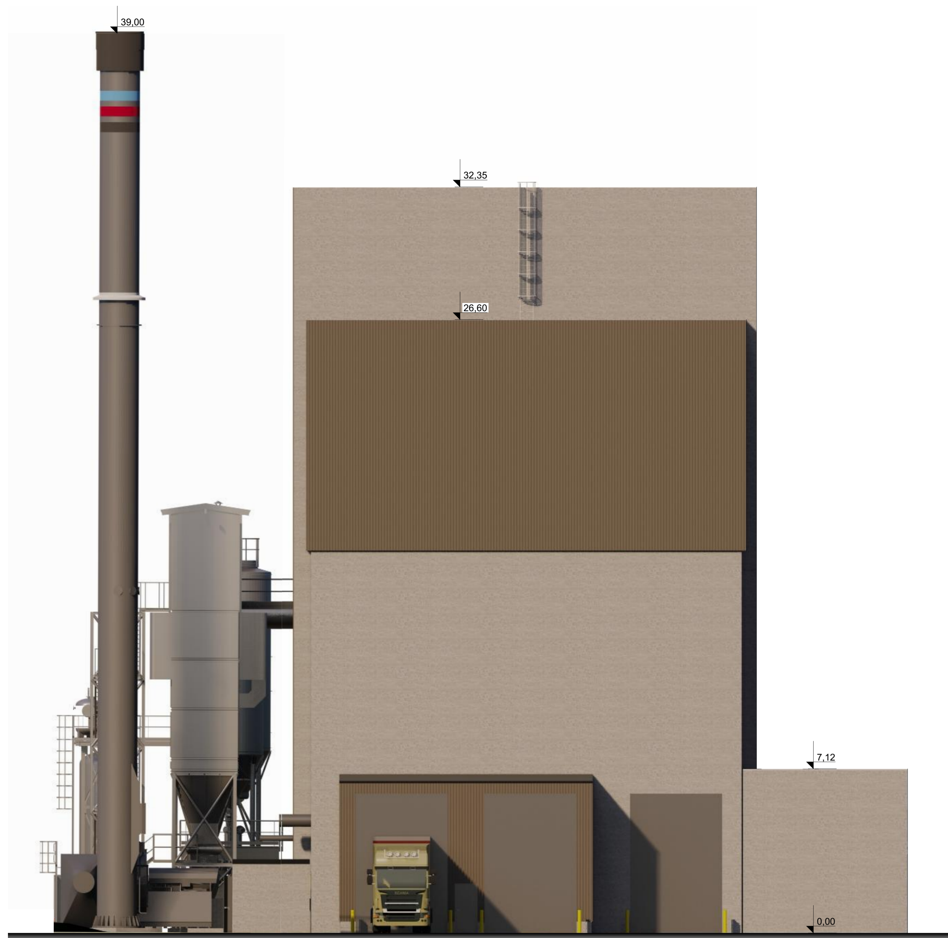
1:100 Façade Est-Chaudière - PC5
