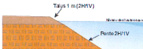
(F) Berges sur remblais
