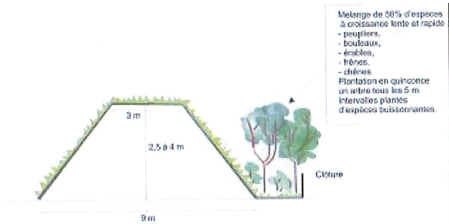
Vue en coupe du merlon (site en exploitation)
