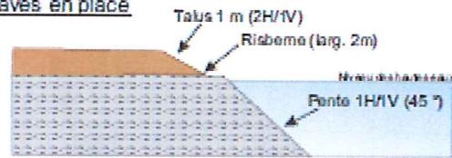
(B) Berges aval sur graves en place
